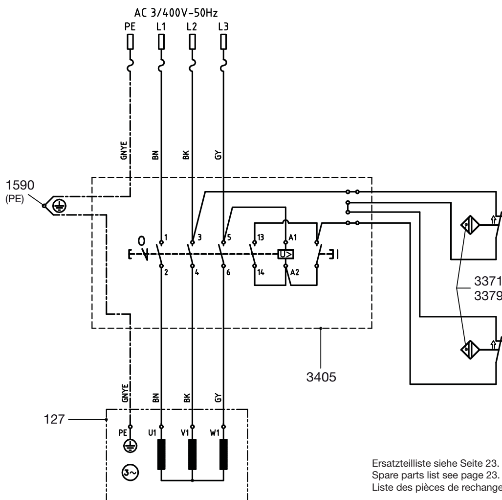
Schéma de câblage élec- trique
